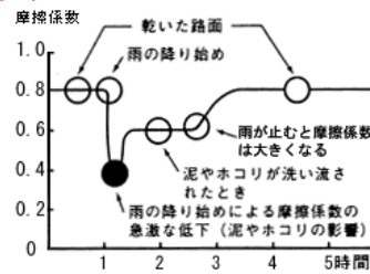
図2:雨による路面の摩擦係数の変化
