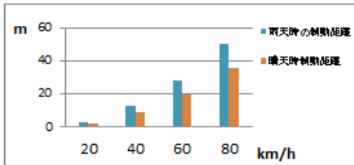
図1:雨天時の制動距離
