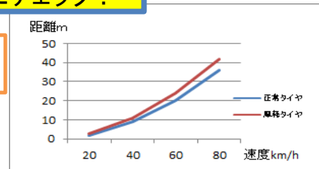
図3:タイヤの状態別制動距離
